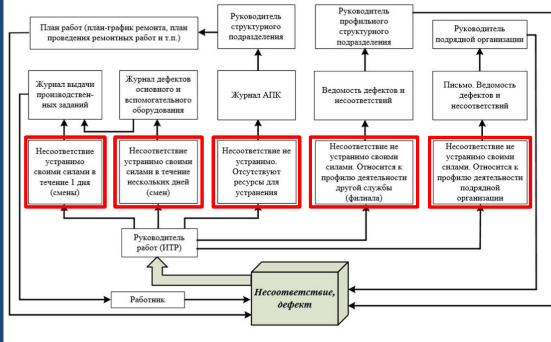
Блок-схема процесса обмена информацией АПК на 1 уровне
